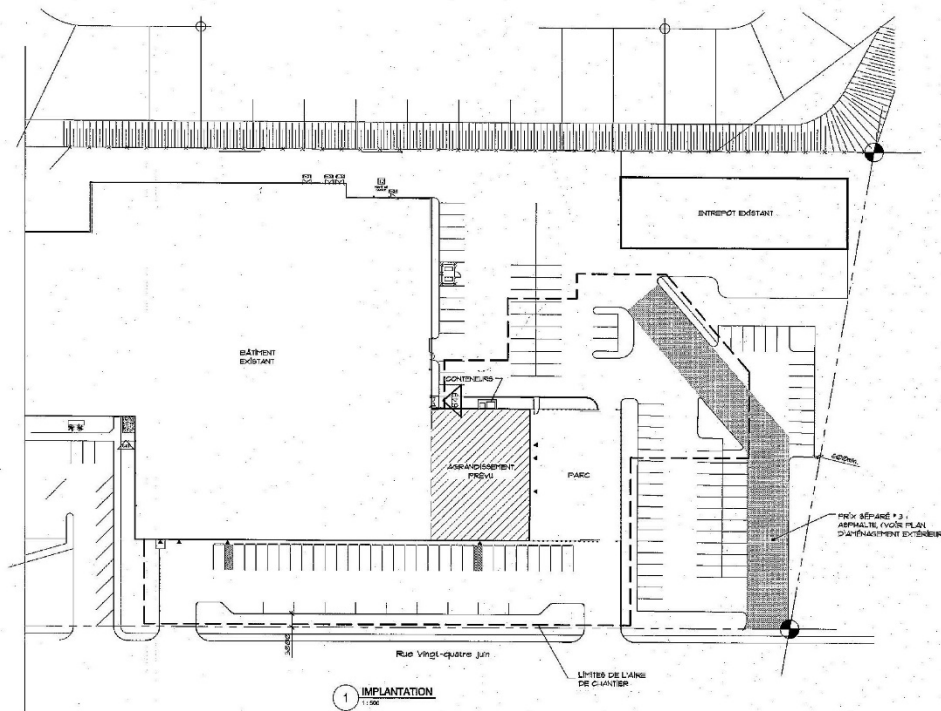
Détail du plan d'implantation de l'agrandissement des ateliers mécaniques, avril 2004. (P-170-013-025, FC.18 Plans des établissements de la CSRS)
