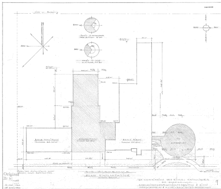
Plan d'implantation préliminaire de l'agrandissement des écoles Biron et Chalifoux, mai 1966. (P-004-002-001, FC.18 Plans des établissements de la CSRS)
