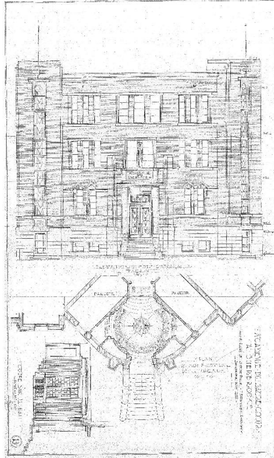
Élévation du motif central de la façade, août 1935. (P-024-001-013, FC.18 Plans des établissements de la CSRS)
