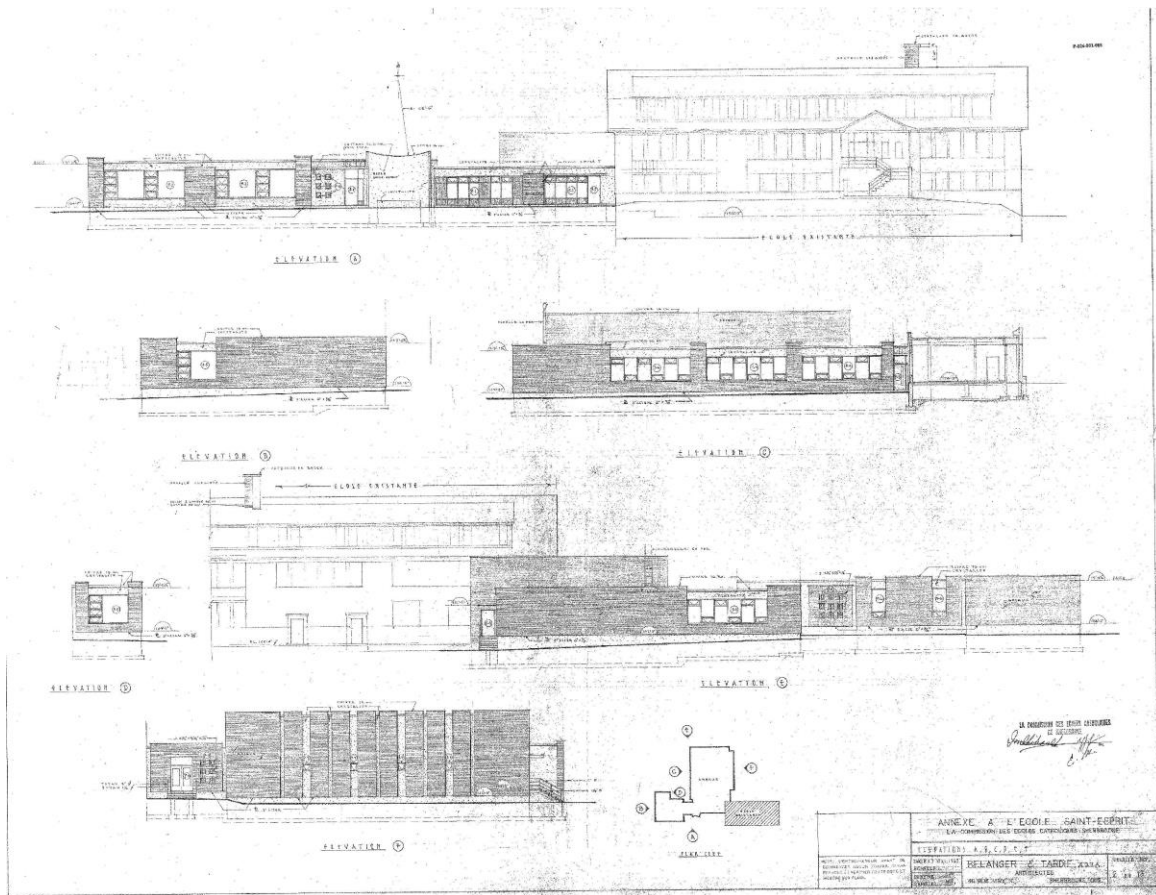
Plan des élévations et d'implantation de l'agrandissement de l'école du Saint-Esprit, mai 1967. (P-026-001-018, FC.18 Plans des établissements de la CSRS)
