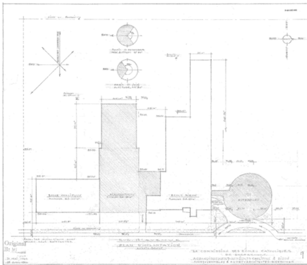
Plan d'implantation préliminaire de l'agrandissement-fusion des écoles Biron et Chalifoux, mai 1966. (P-004-002-001, FC.18 Plans des établissements de la CSRS)
