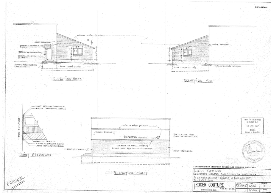
Plan des élévations Nord, Sud et Ouest concernant l'ajout de rangement à l'extrémité du gymnase, mars 1997. (P-034-002-001, FC.18 Plans des établissements de la CSRS)
