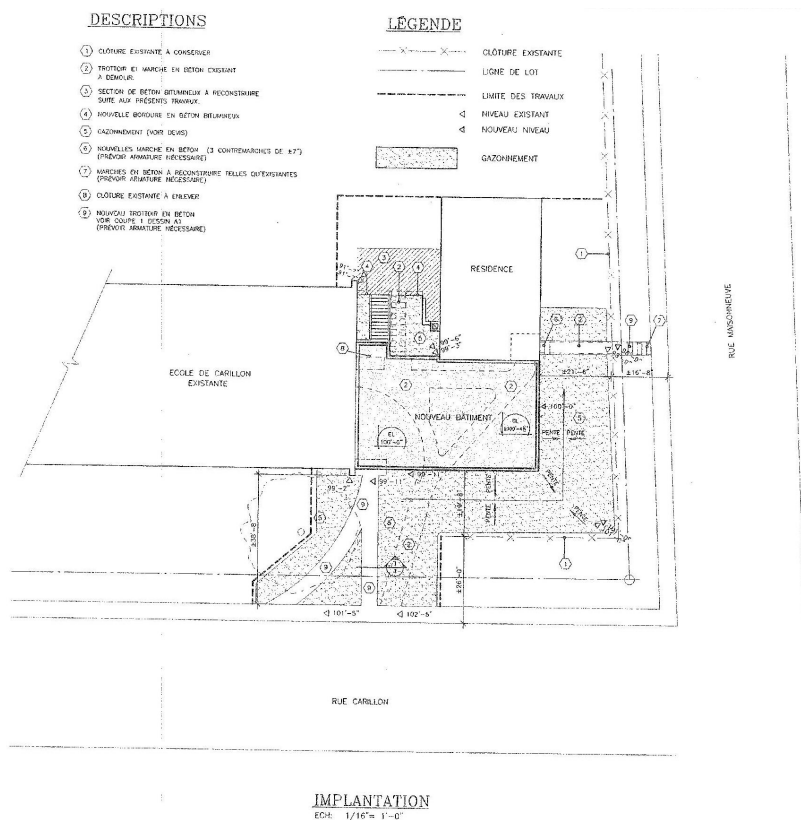
Détail du plan d'implantation du local polyvalent, juin 2000. (P-034-002-014, FC.18 Plans des établissements de la CSRS)
