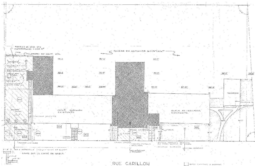
Détail du plan d'implantation de la construction jumelant les écoles Saint-Boniface et de Carillon, février 1966. (P-034-001-008, FC.18 Plans des établissements de la CSRS)
