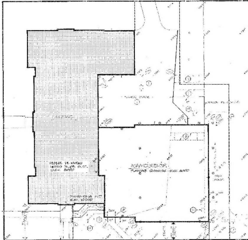
Détail du plan d'implantation du gymnase, juin 1989 (tel que construit). (P-013-001-051, FC.18 Plans des établissements de la CSRS )
