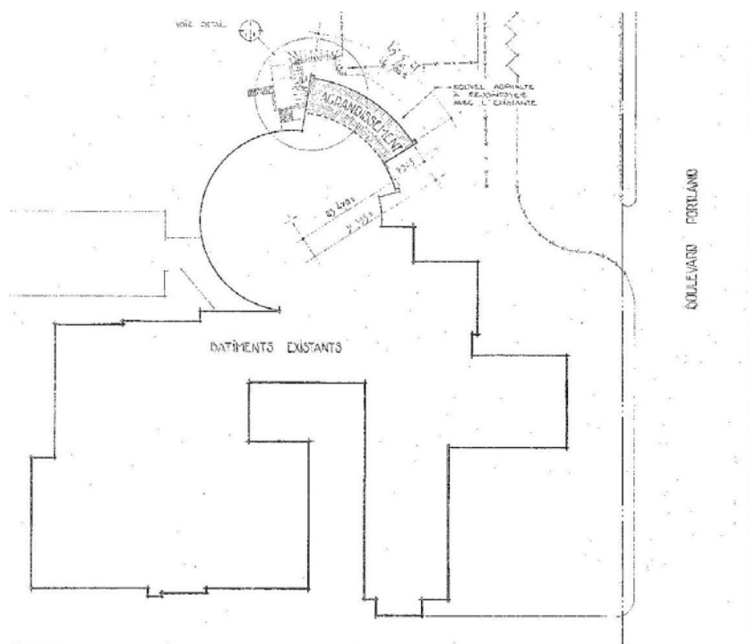
Détail du plan d'implantation de l'agrandissement de la cafétéria de l'école Montcalm, 1982 (tel que construit). (P-124-004-029, FC.18 Plans des établissements de la CSRS)
