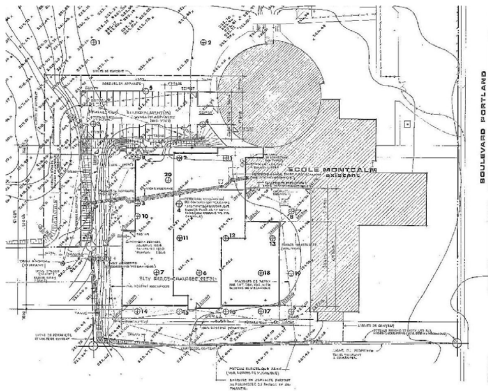
Détail du plan d'implantation de l'agrandissement de l'école Montcalm, décembre 1978. (P-124-003-002, FC.18 Plans des établissements de la CSRS)
