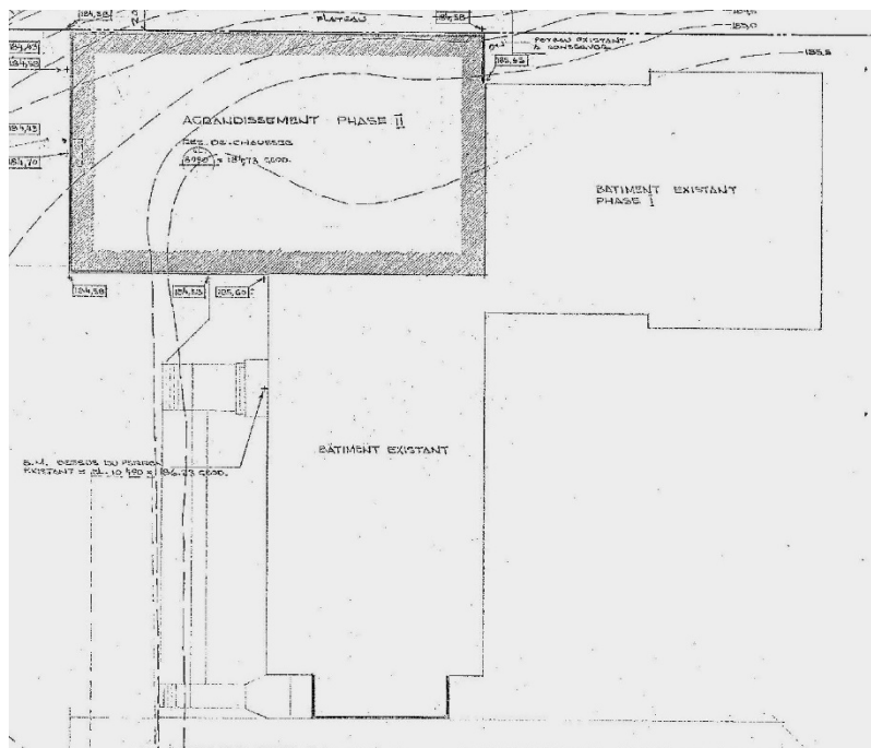
Détail du plan d'implantation de la phase II d'agrandissement, décembre 1987 (tel que construit). (P-037-001-046, FC.18 Plans des établissements de la CSRS)
