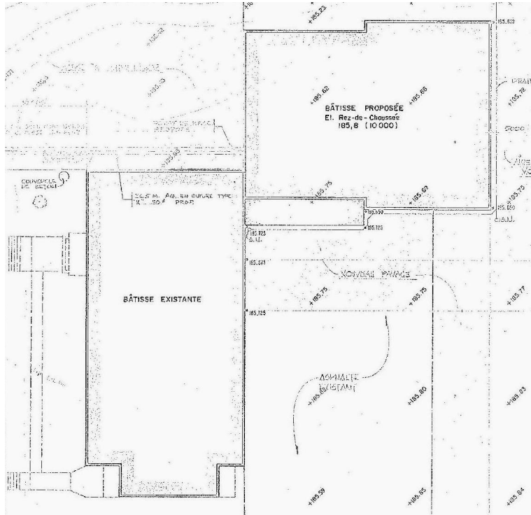
Détail du plan d'implantation de la phase I d'agrandissement, mai 1984. (P-037-001-011, FC.18 Plans des établissements de la CSRS)
