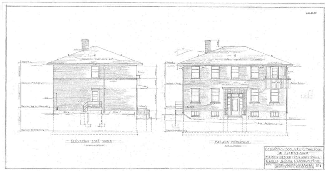
Plan des élévations Nord et Ouest de la résidence des sœurs de l'école de l'Assomption, été 1956. (P-011-001-003, FC.18 Plans des établissements de la CSRS)
