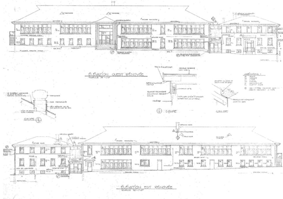
Détail du plan des élévations Ouest et Est relatif au réaménagement de l'école de l'Assomption, mai 1991. (P-011-001-043, FC.18 Plans des établissements de la CSRS)
