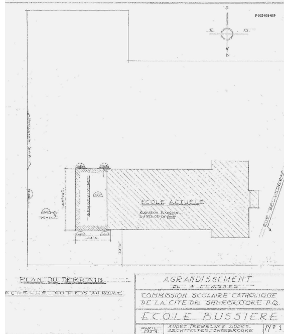
Détail du plan d'implantation de l'agrandissement de l'école Bussière, avril 1959. (P-002-001-019, FC.18 Plans des établissements de la CSRS)
