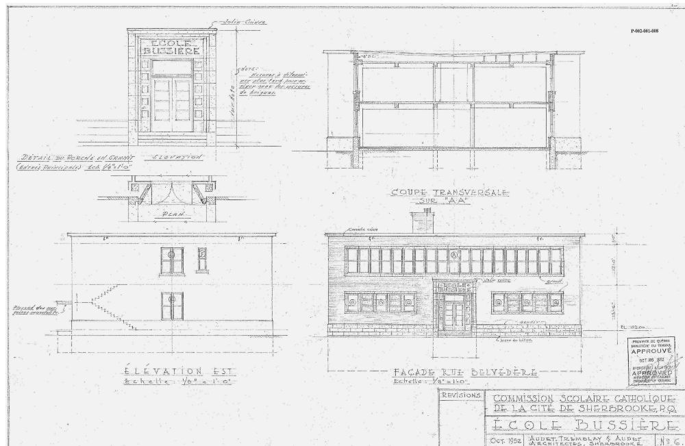
Plans relatifs à la construction de l'école Bussière, octobre 1952. (P-002-001-008, FC.18 Plans des établissements de la CSRS)
