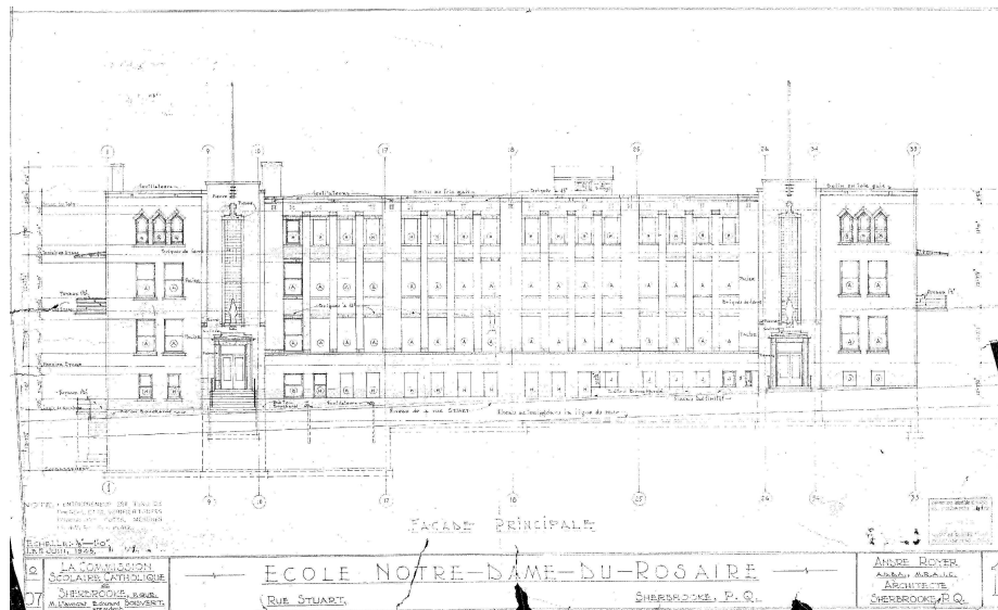
Plan de la façade principale de l'école Notre-Dame-du-Rosaire, juin 1945. (P-021-001-001, FC.18 Plans des établissements de la CSRS)
